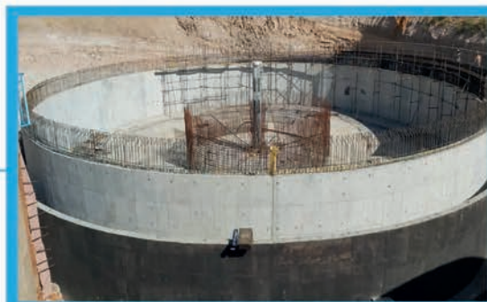
احداث مخزن زلال‌ساز تصفیه‌خانه آب مراغه ■ شروع عملیات از سال ۱۳۹۹ و در حال اجرا ■ ظرفیت: ۵ هزار متر مکعب ■ اعتبار: ۱۵۰ میلیارد ریال
